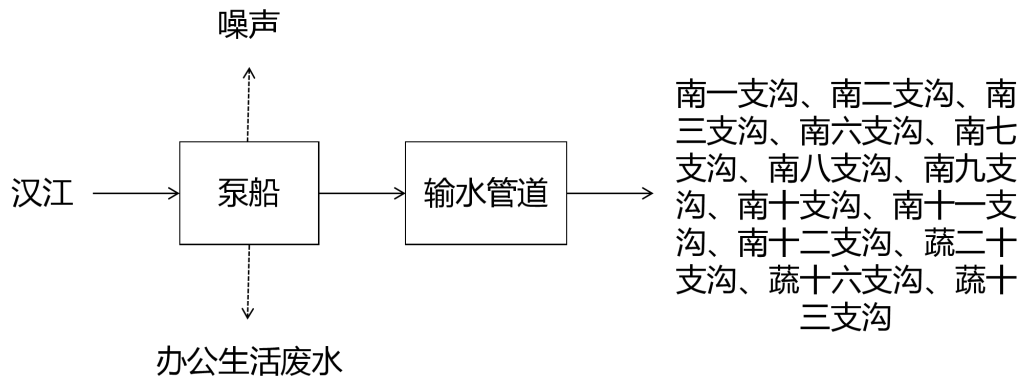
图 4.3-3 取水工艺流程图
