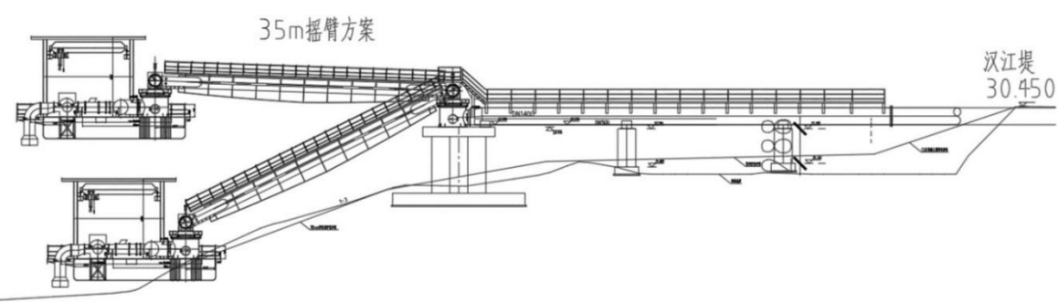
图 3.3-1 摇臂式刚性输水钢管连接+缆绳锚固连接方式剖面布置
