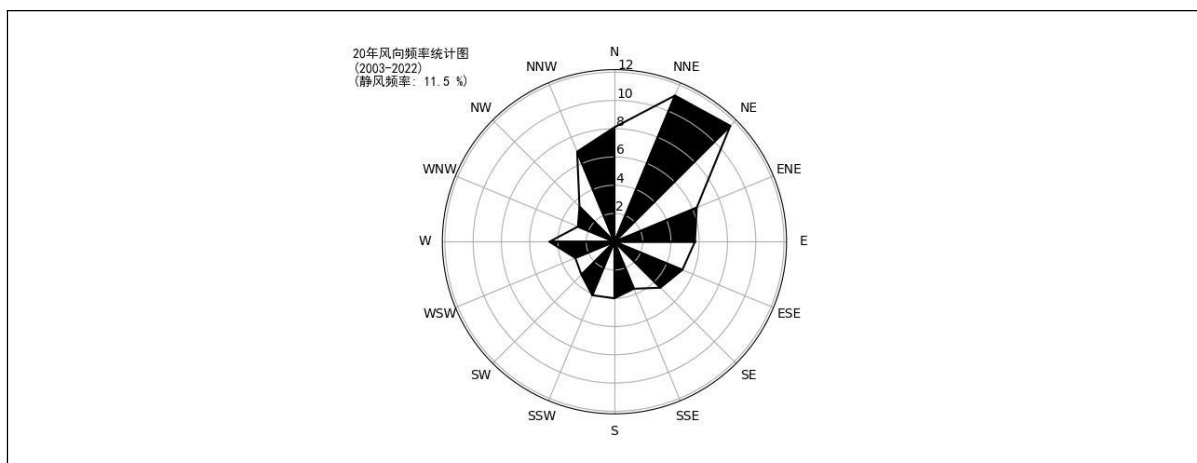
图 5.1-1 武汉市近 20 年平均风向玫瑰图
