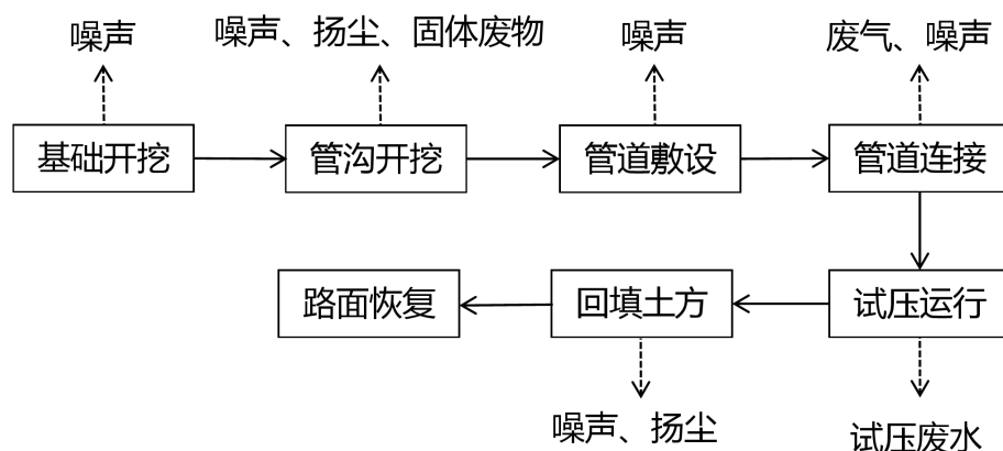
图 4.3-1 管道施工工艺流程及产污环节图
