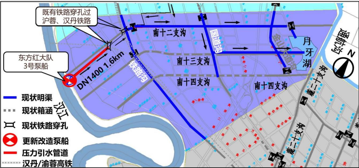
图 3.3-3 东方红泵船引水压力管道完善总体布置图
