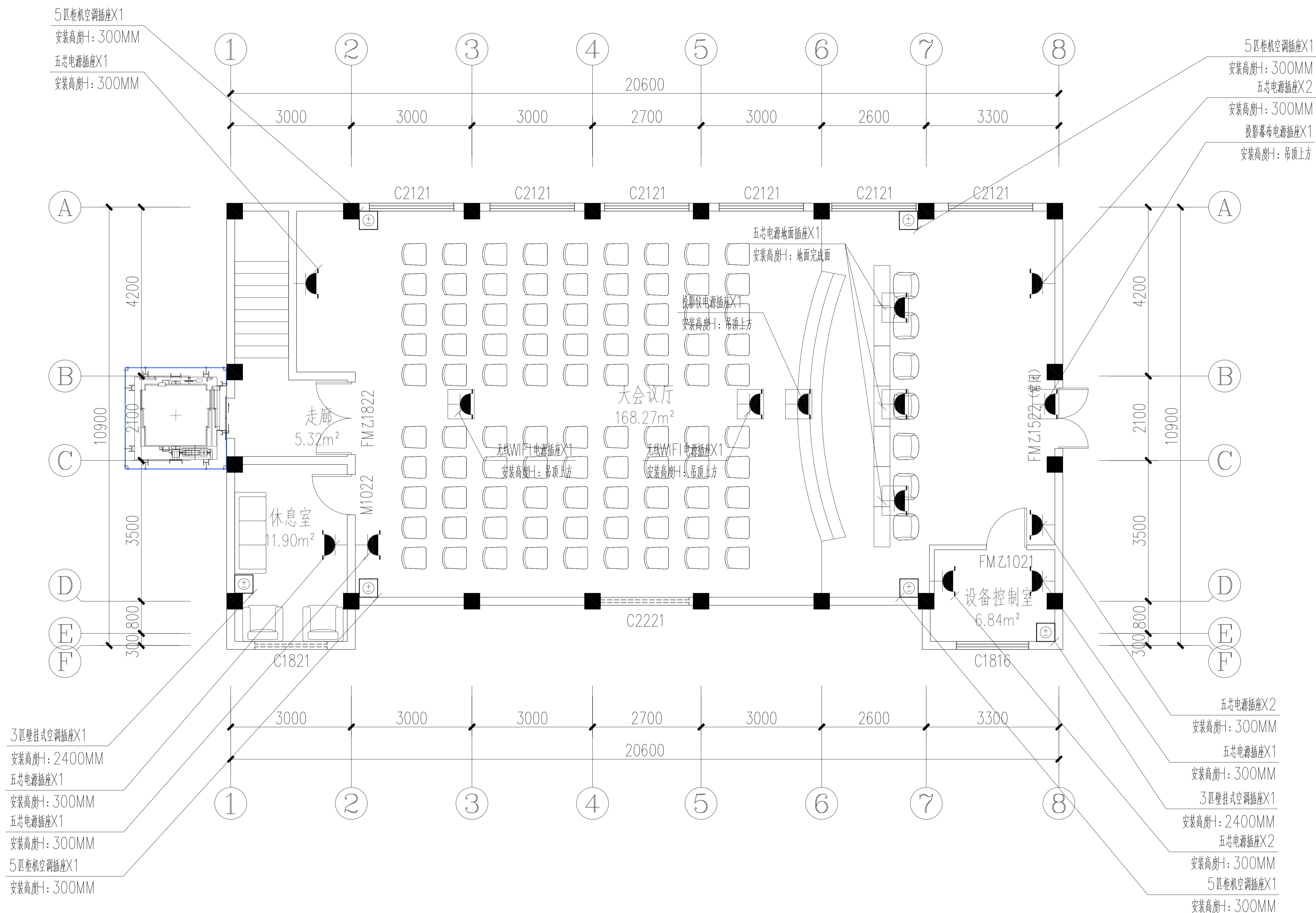
FF-7F FURNITURE 七层强电插座布置图 Scale 1:50
