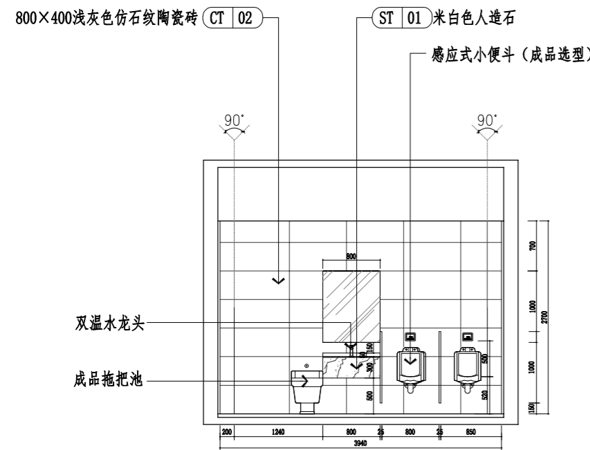
E ELEVATION 1N-3F 男卫生间E立面图 SCALE 1:50
