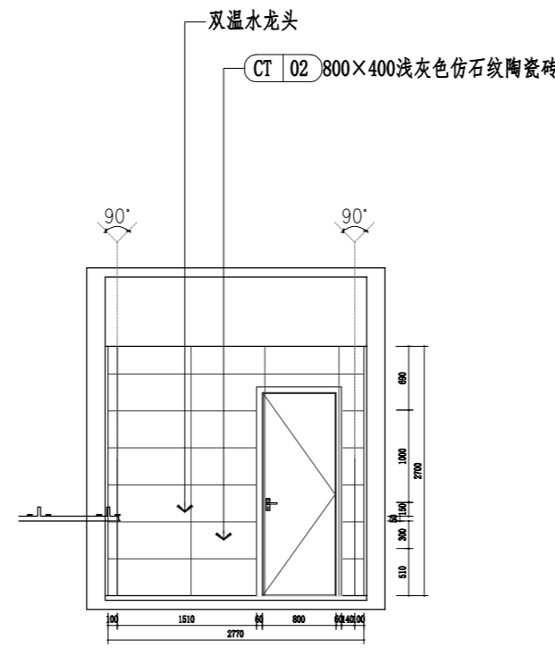
B ELEVATION 1N-2F 女卫生间B立面图 SCALE 1:50
