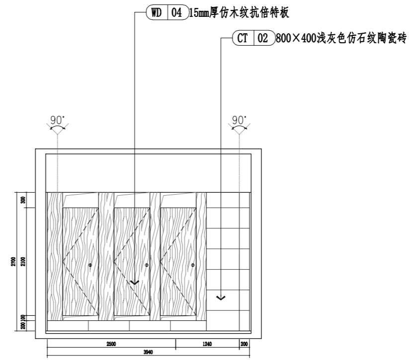
C ELEVATION 1N-2F 女卫生间C立面图 SCALE 1:50
