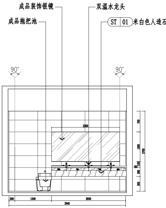
A ELEVATION 1N-2F 女卫生间A立面图 SCALE 1:50
