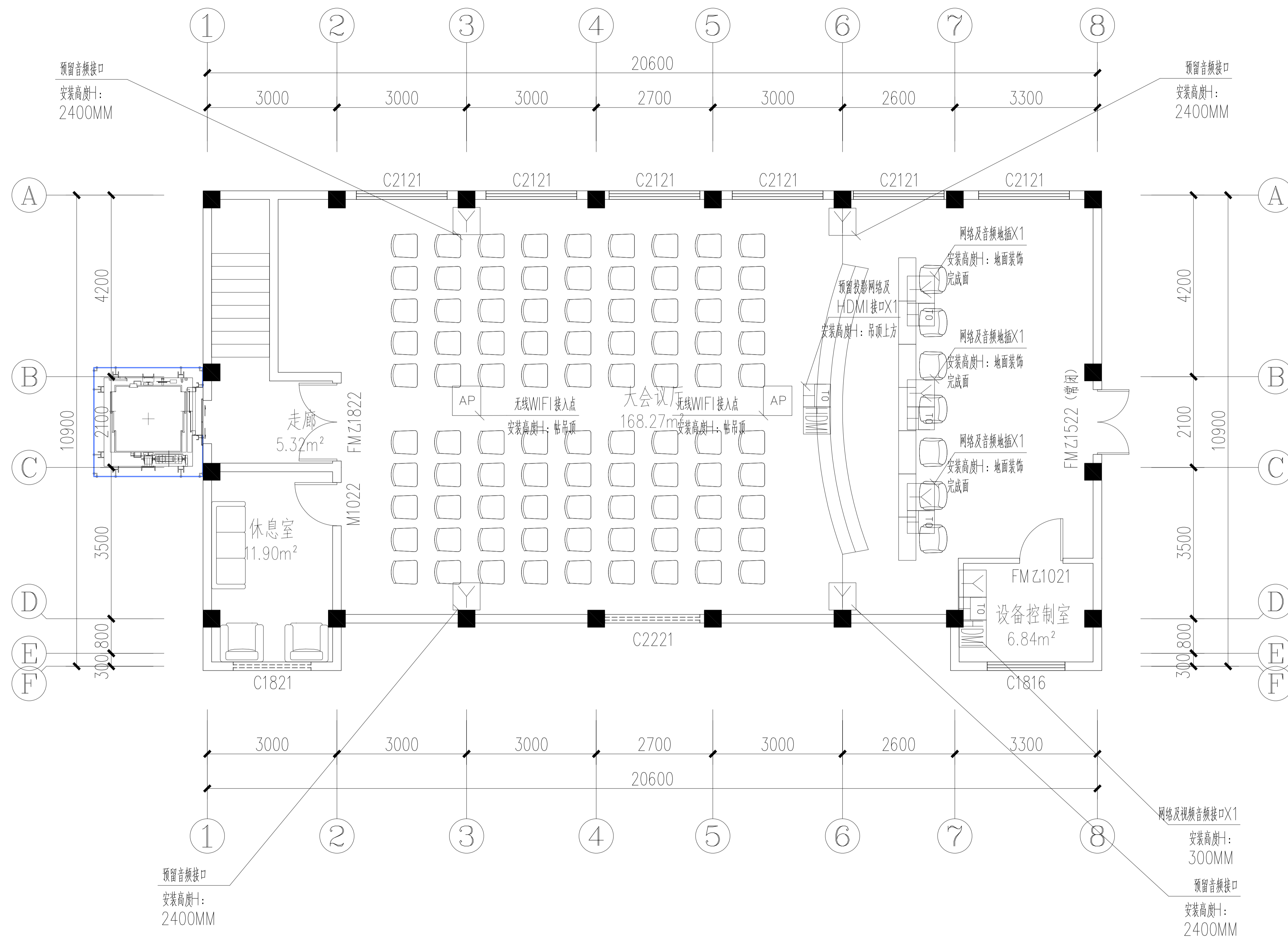
FF-7F FURNITURE 七层弱电插座布置图 Scale 1:50
