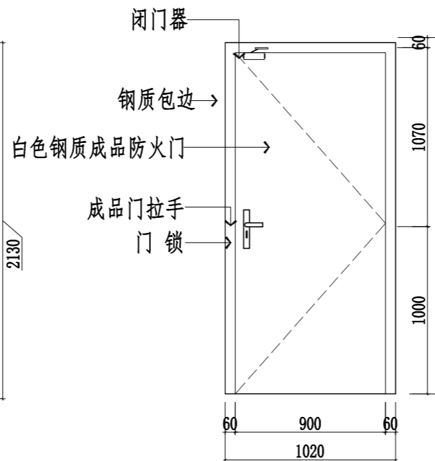
FM乙1021
