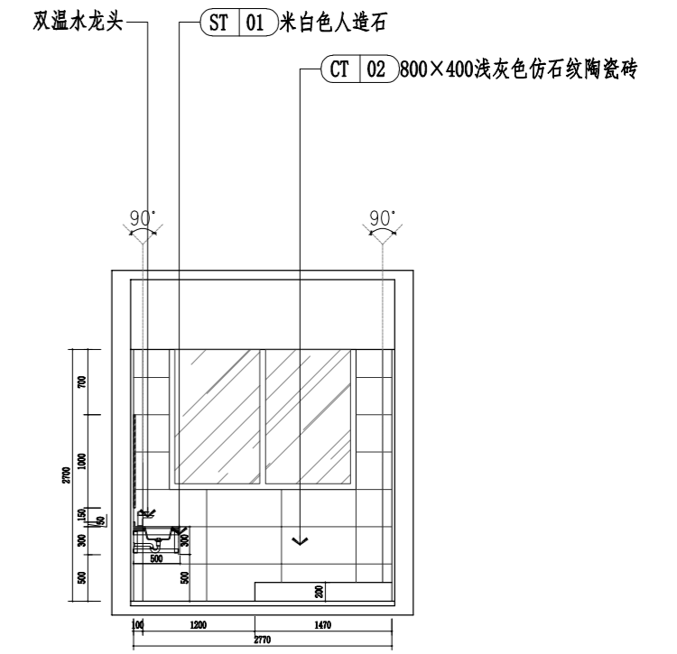
D ELEVATION 1N-2F 女卫生间D立面图 SCALE 1:50
