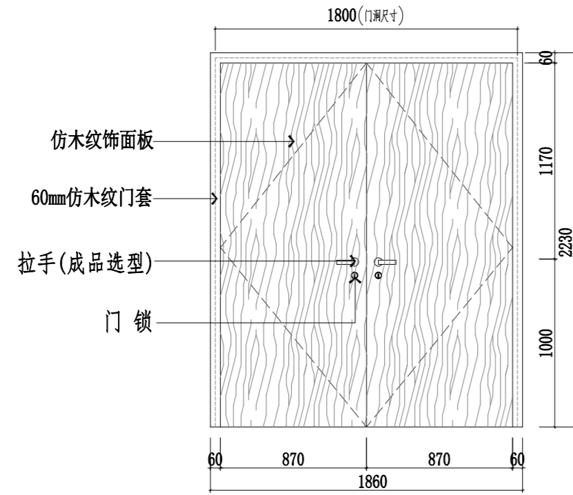
FM乙1821
