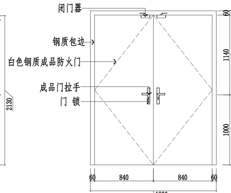
FM乙1822
