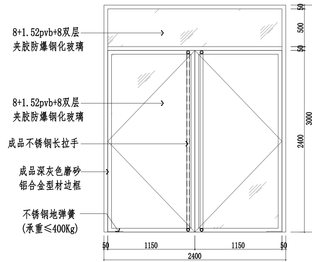
GM2424a
