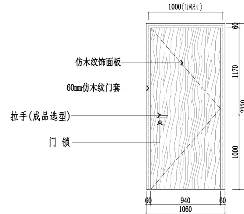
M1022
