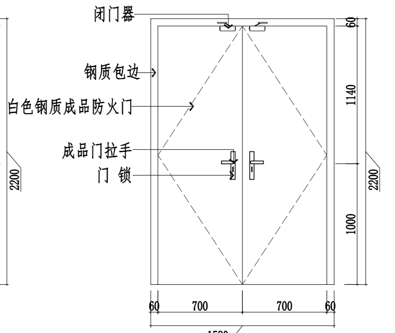
FM乙1522 (常闭)
