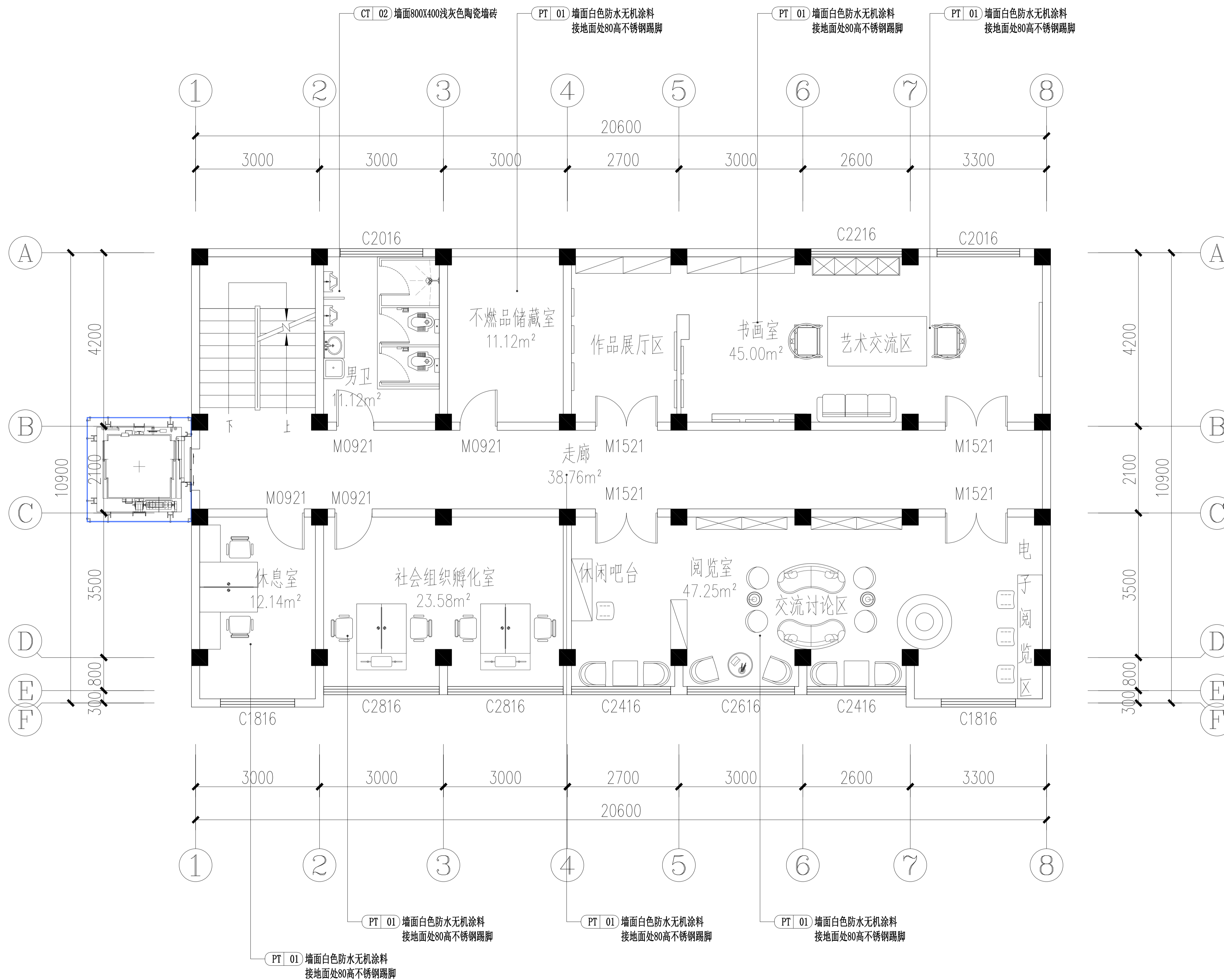
F1-3F FACADE INDEX 三层材料标志图 Scale 1:50
