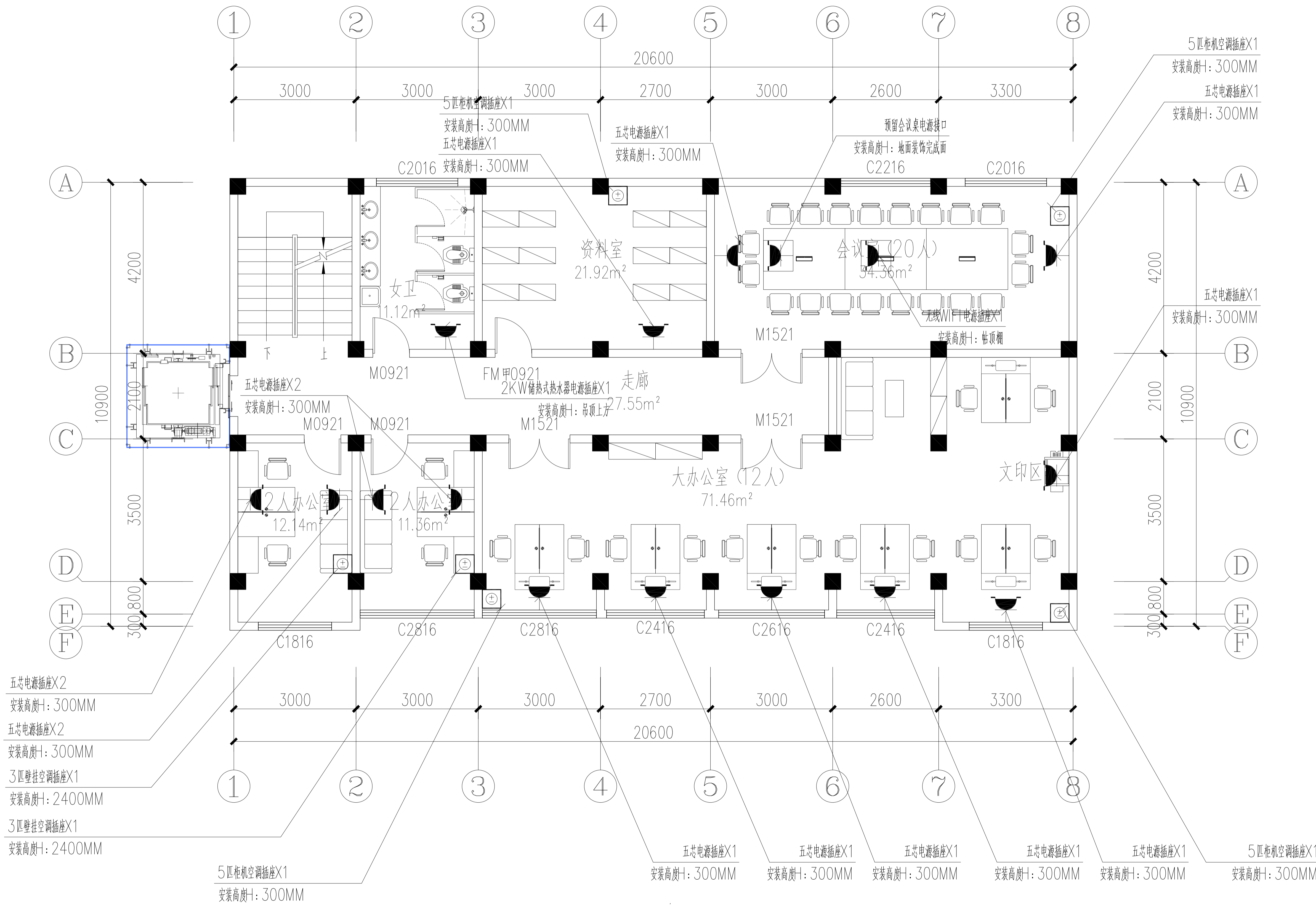
EP-2F FACADE INDEX 二层强电插座布置图 Scale 1: 50
