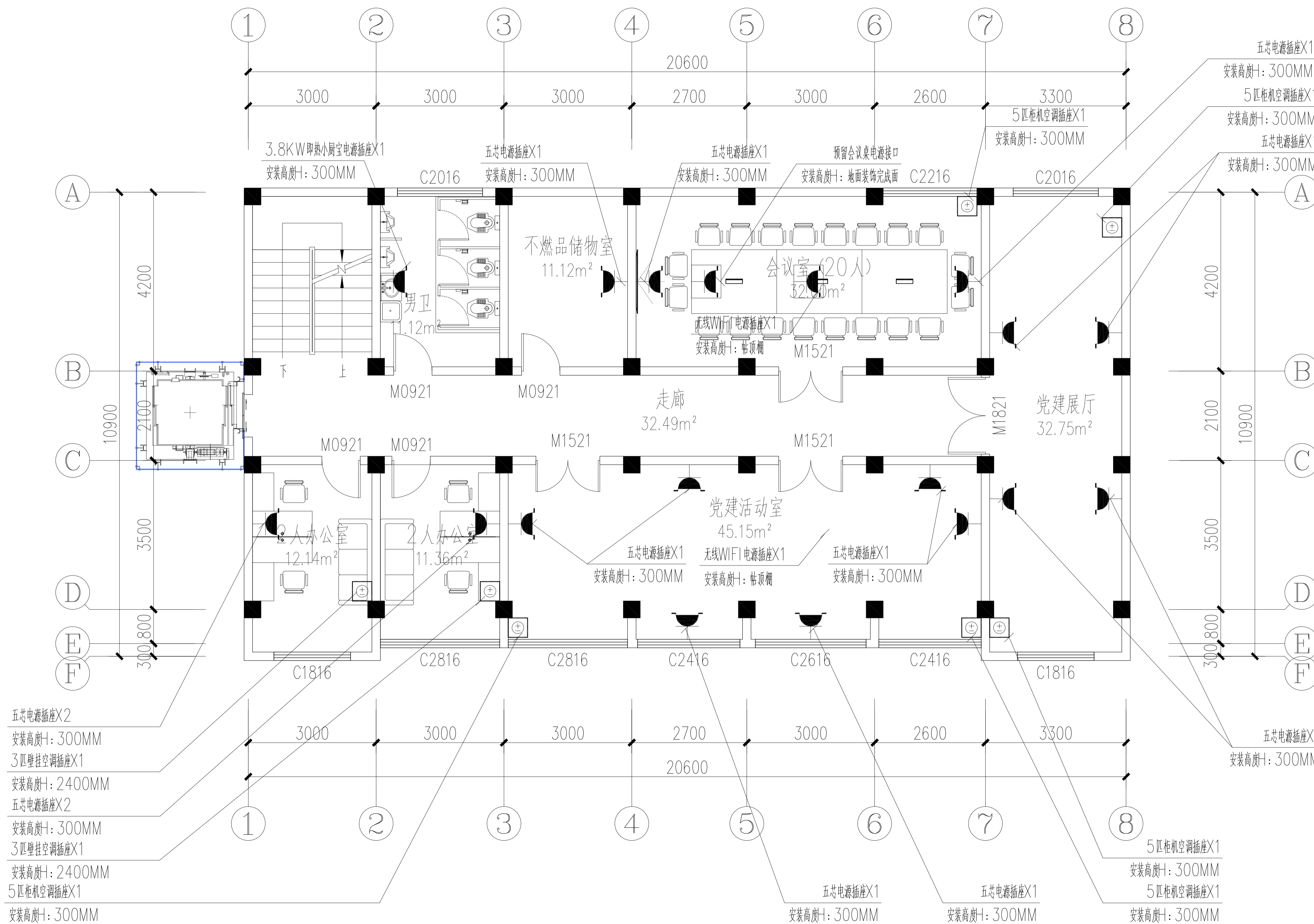
FF-5F FURNITURE 五层强电插座布置图 Scale 1:50
