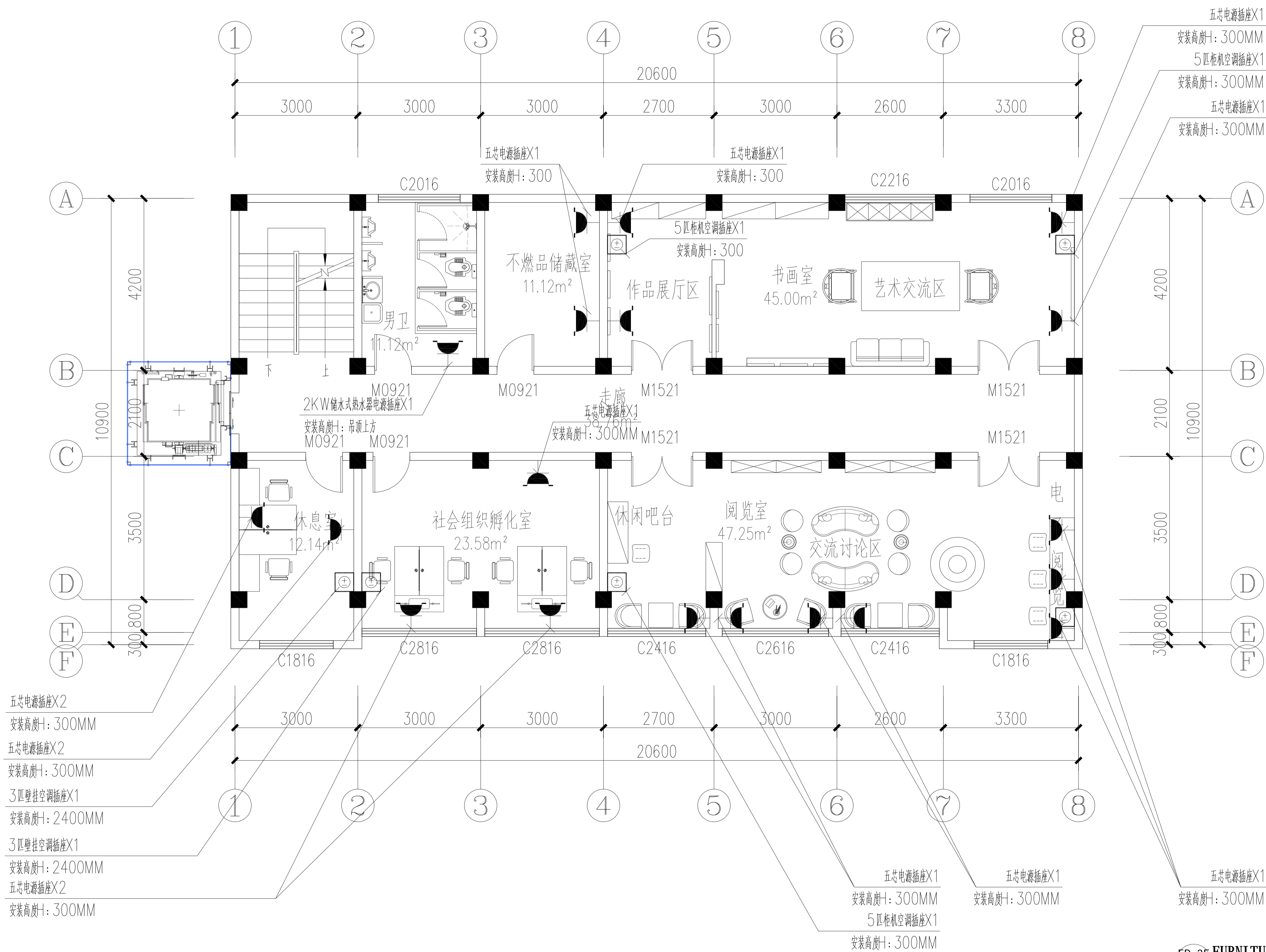
EP-3F FURNITURE 三层强电插座布置图 Scale 1:50
