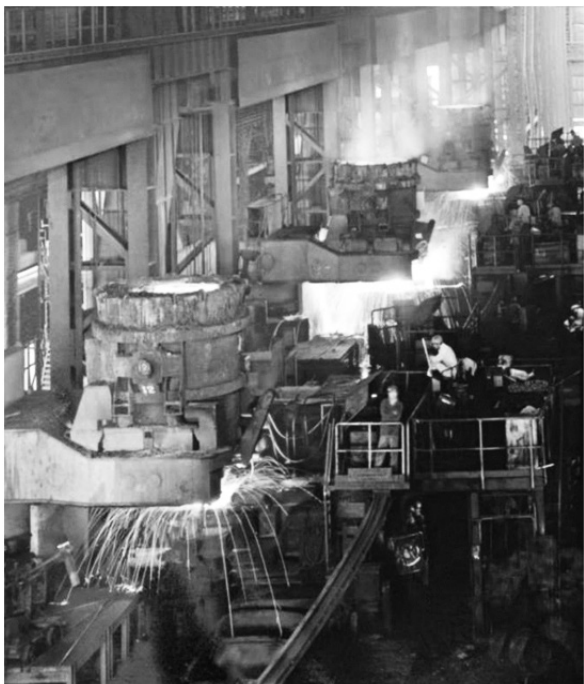
二炼钢厂连铸车间生产线
